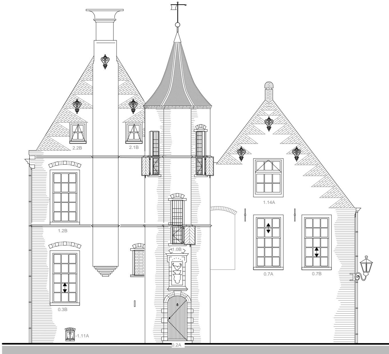
WESTGEVEL
