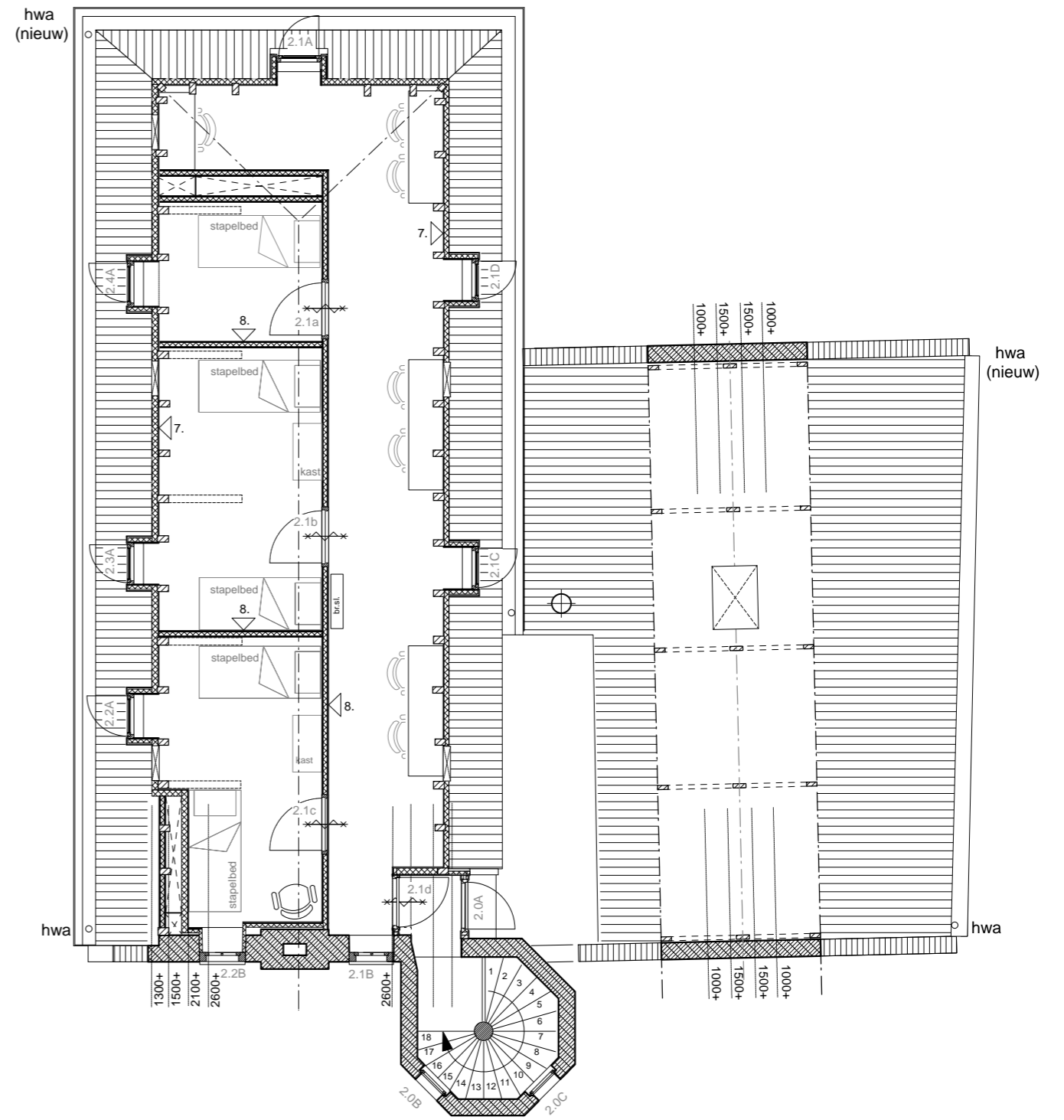
PLATTEGROND ZOLDER
