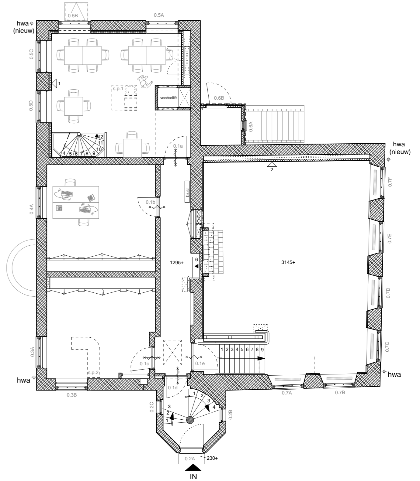
PLATTEGROND BEGANEGROND
