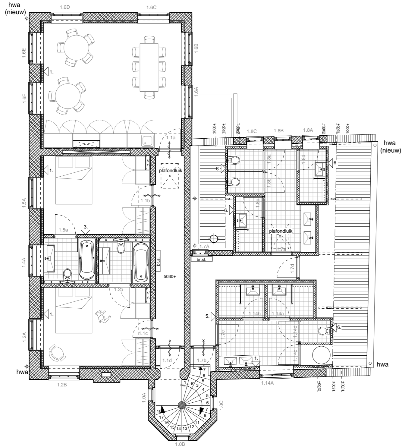
PLATTEGROND VERDIEPING
