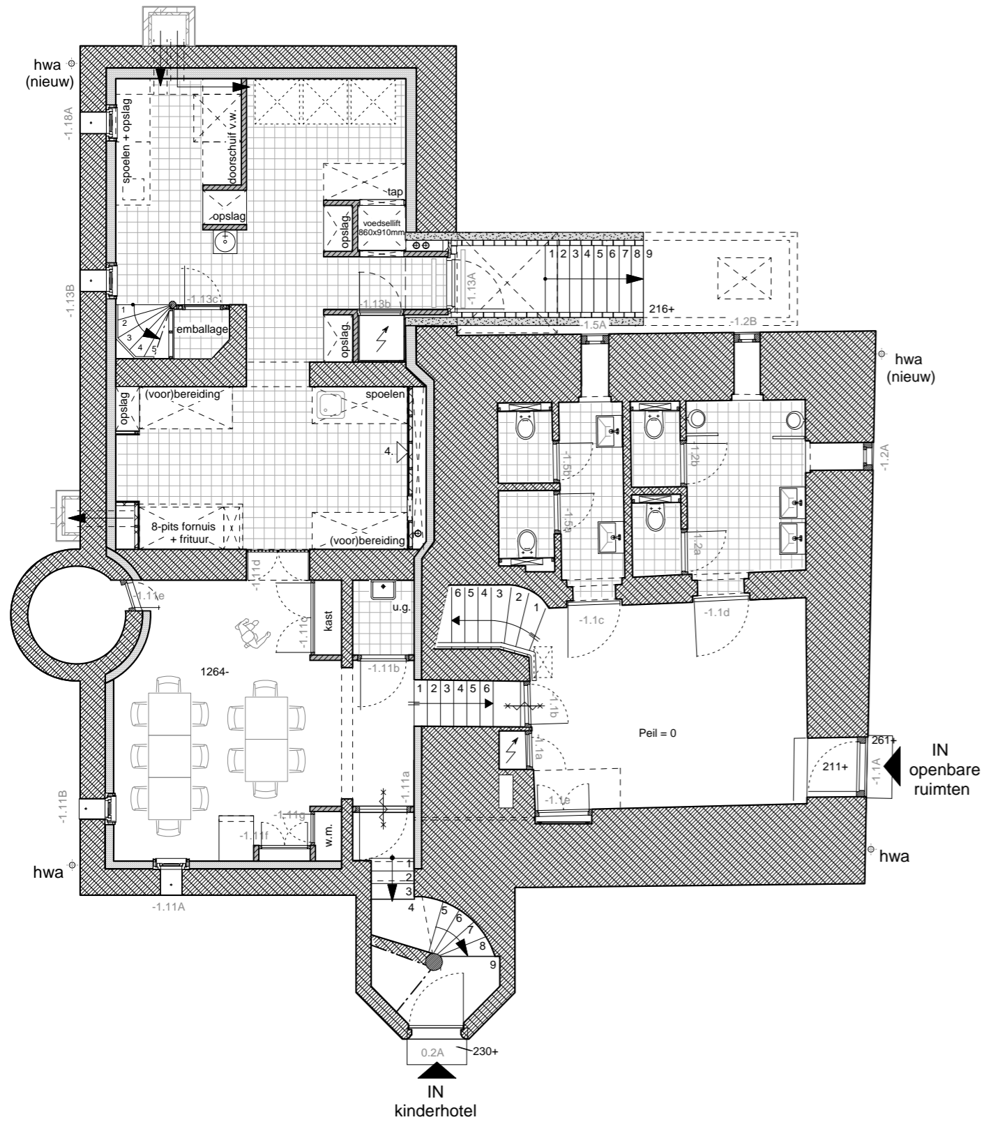
PLATTEGROND SOUTERRAIN
