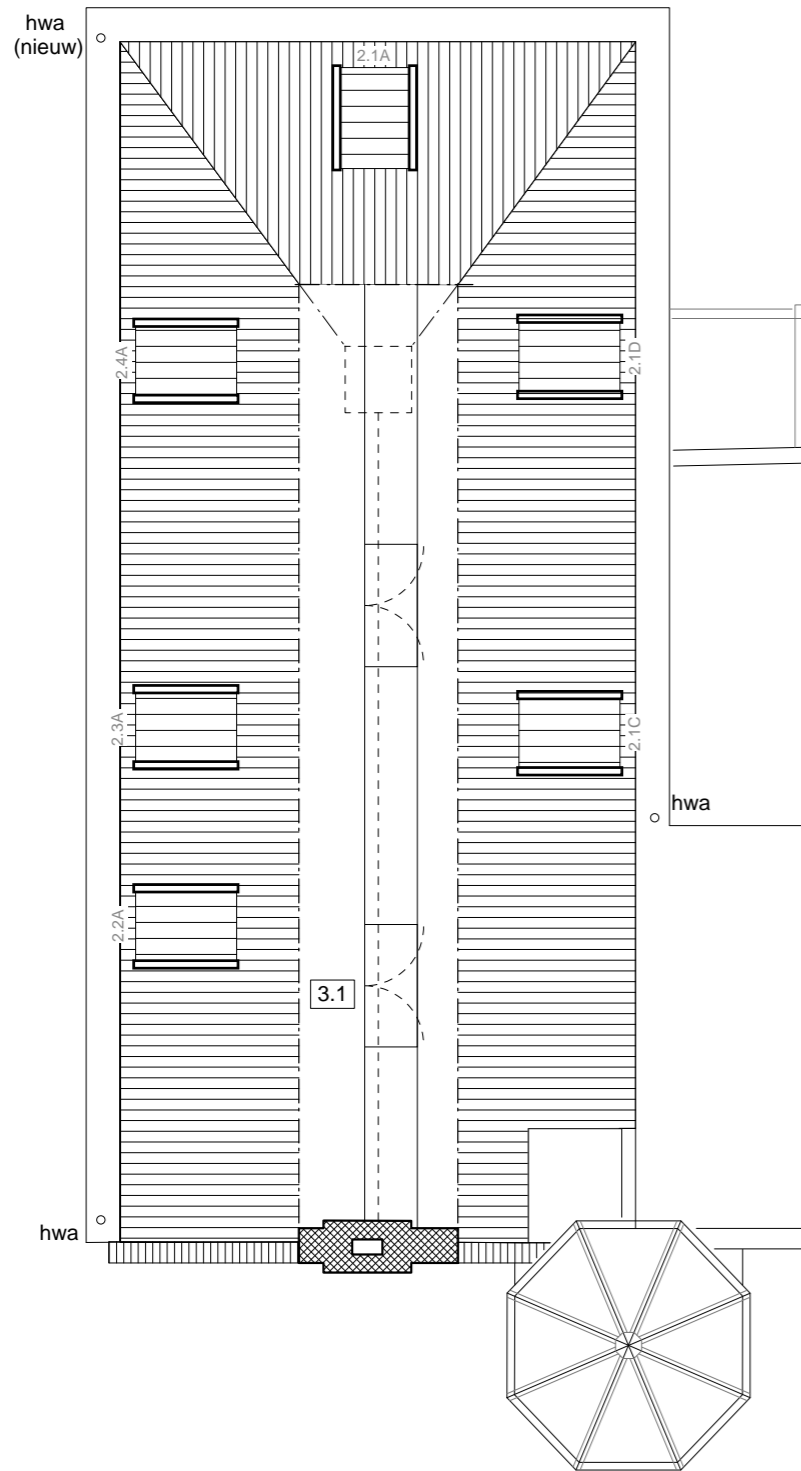
PLATTEGROND VLIERING
