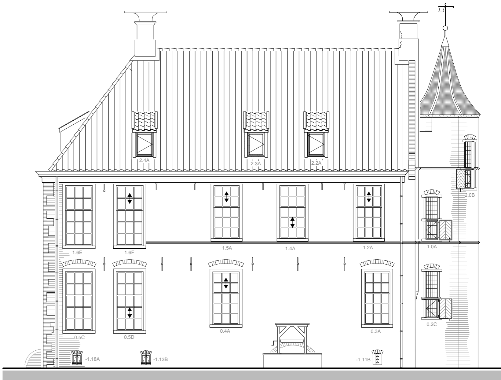
NOORDGEVEL
