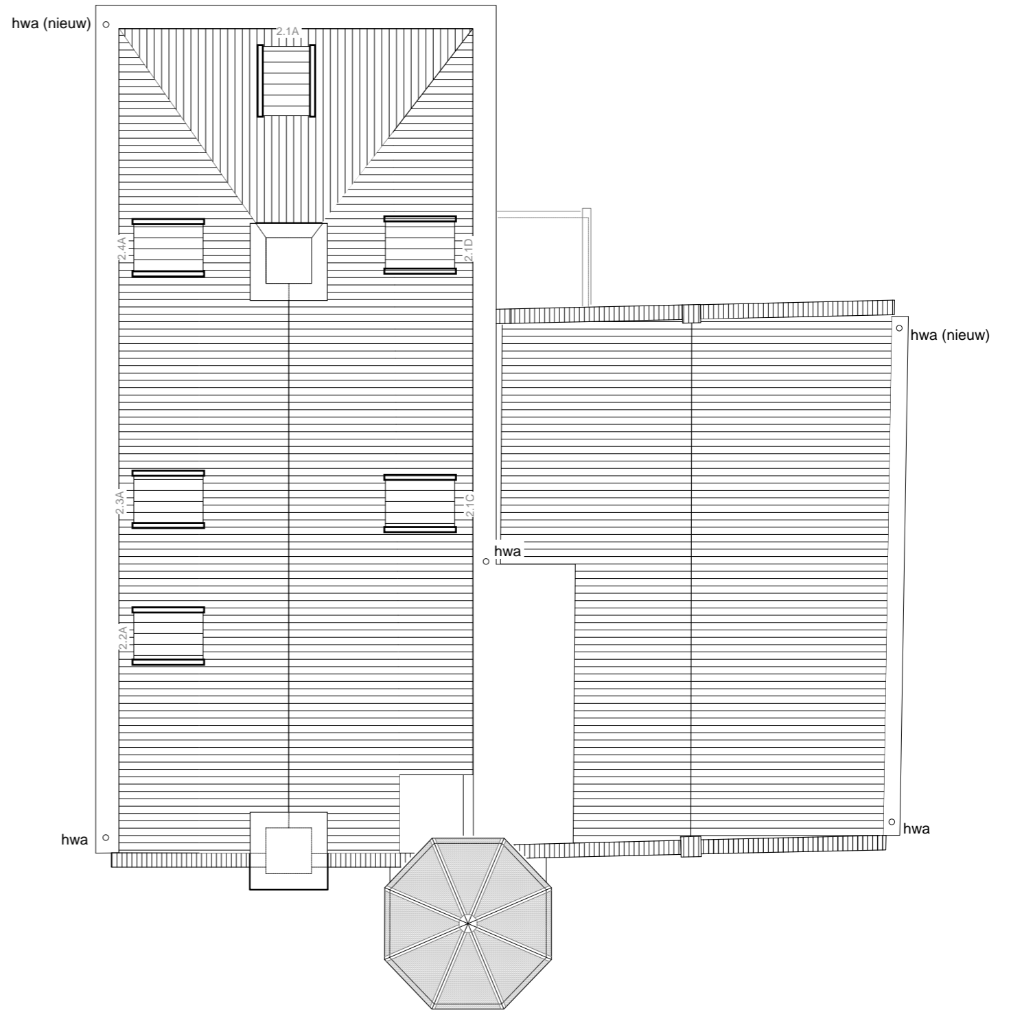
DAKOVERZICHT
