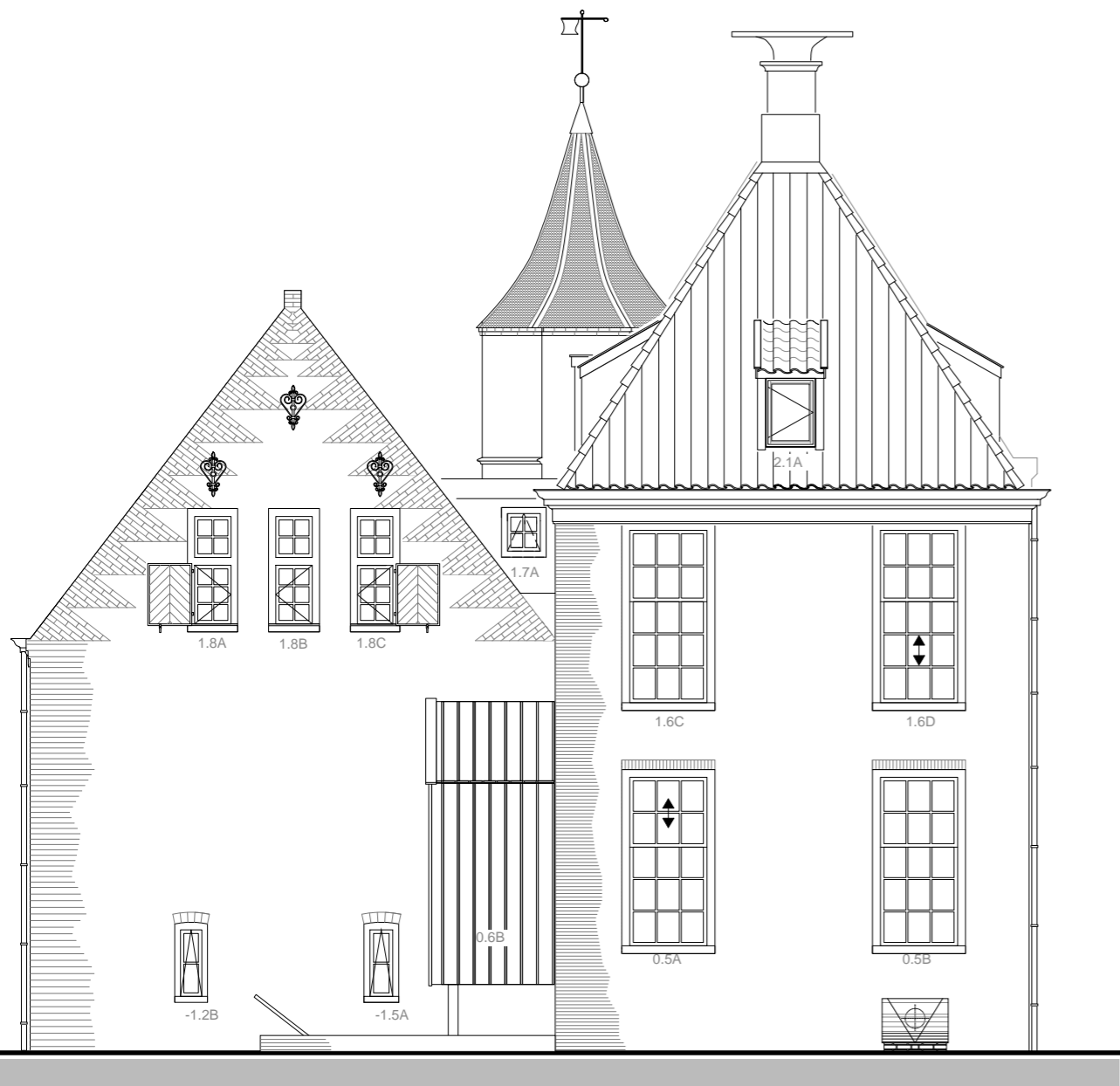
OOSTGEVEL
